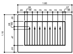
Balcon de Ventana Tipo V-1 METAL 2 Unidad
