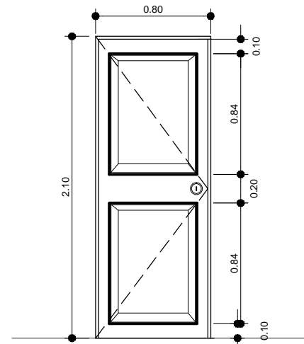
Puerta Tipo P-6
