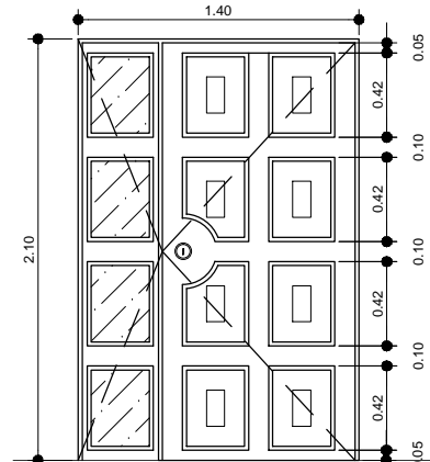
Puerta Tipo P-2
