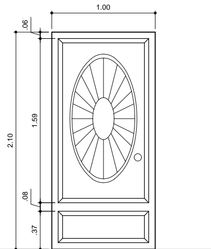
Puerta Tipo P-10
