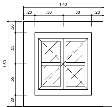
Ventana Tipo V-2
