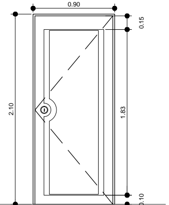
Puerta Tipo P-3
