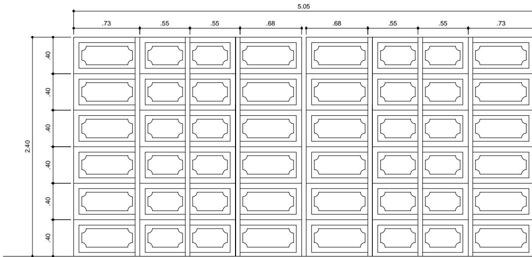
Puerta Tipo P-1
