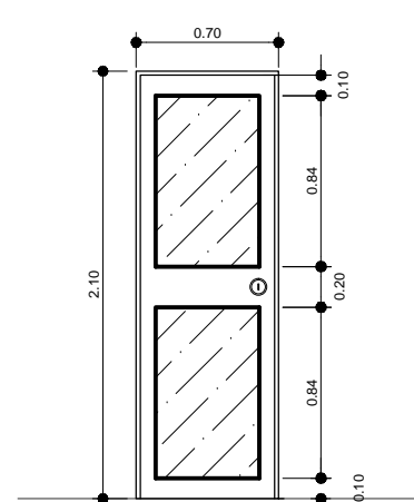
Puerta Tipo P-7
