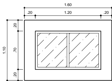
Ventana Tipo V-1
