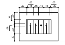
Balcon de Ventana Tipo V-10 METAL 2 Unidad
