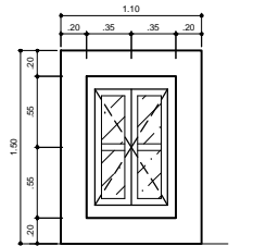
Ventana Tipo V-4 Aluminio 2 Unidad
