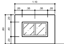
Ventana Tipo V-10 Aluminio 2 Unidad
