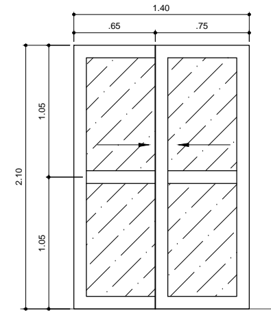
Puerta Tipo P-8
