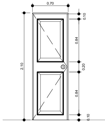
Puerta Tipo P-4
