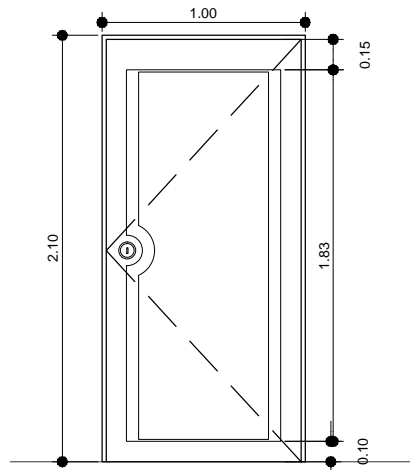
Puerta Tipo P-5
