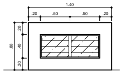
Ventana Tipo V-5 Aluminio 4 Unidades
