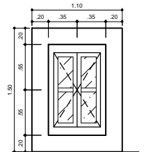
Ventana Tipo V-9 Aluminio 1 Unidad
