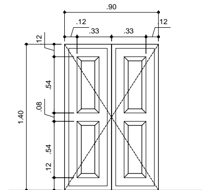
Puerta Tipo P-11
