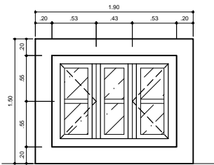
Ventana Tipo V-3 Aluminio 1 Unidad
