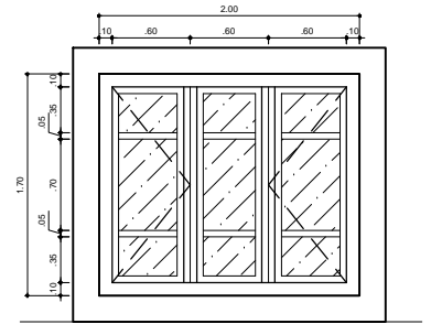
Ventana Tipo V-8 Aluminio 1 Unidades
