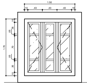
Ventana Tipo V-6 Aluminio 2 Unidades
